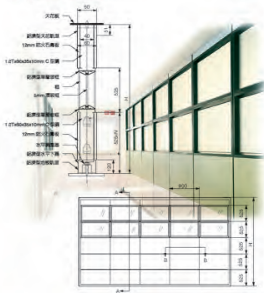
A-A 單層玻璃剖面圖
